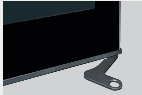
Griff geöffnet
